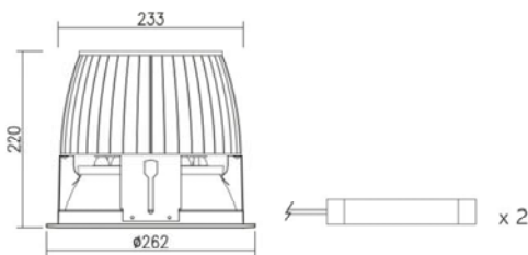
Technische Zeichnung
